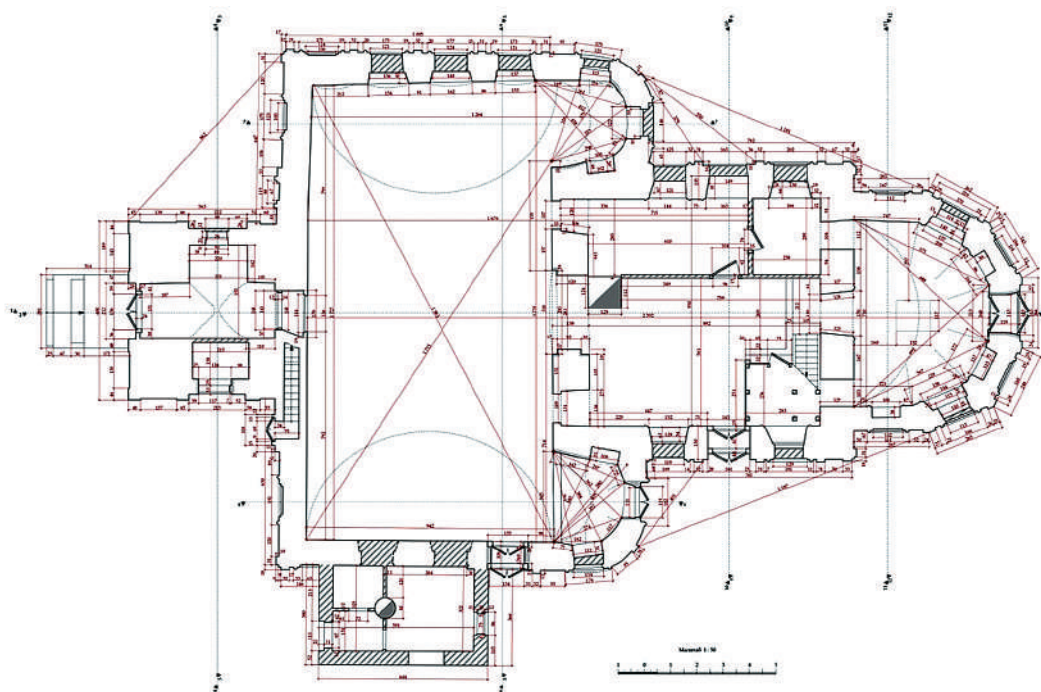
Церковь Рождества Богородицы. Обмерный чертеж. План на отм. 0.000.
